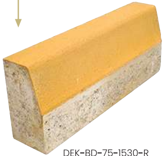
DEK-BD-75-1530-R Karayolları Bordürü 68 kg /Palette 18 adet Palet Ağırlığı : 1.224 kg
