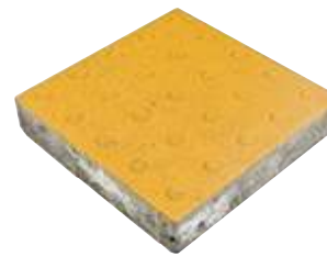
DEK-ET-001-R Engelli Taşı 30 kg /Palette 90 adet Palet Ağırlığı : 2.700 kg
